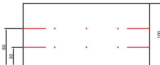
Vue de face gabion 200x50x100 cm
