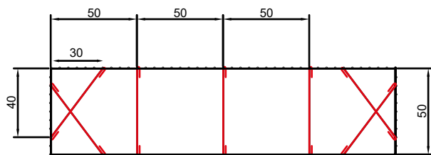
Vue de dessus gabion 200x50x100 cm
