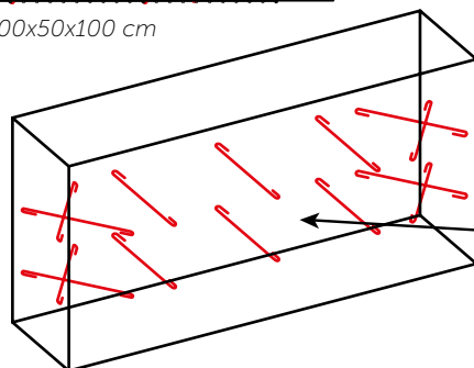
200x50x100 cm gabion vue en perspective
